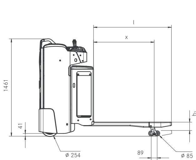
Seitenansicht FXH N
