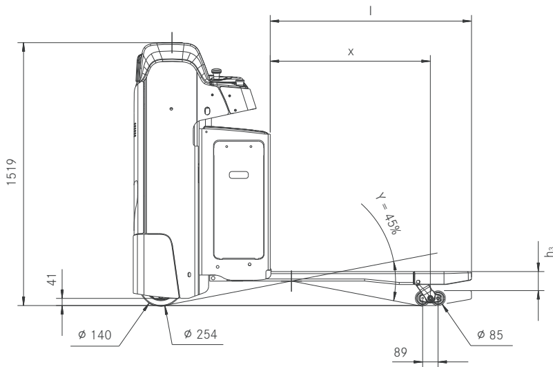
Seitenansicht SXH mit angehobenem Initialhub
