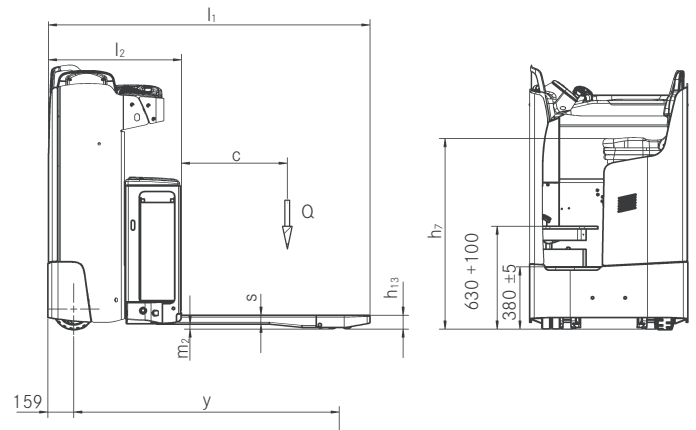
Seitenansicht FXH
