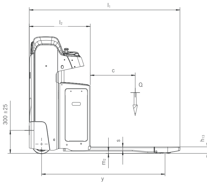
Seitenansicht SXH
